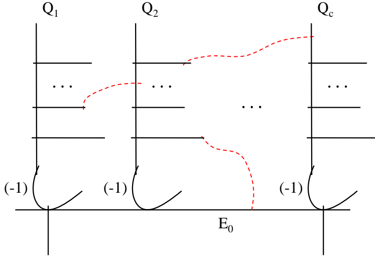
RYSUNEK 1. Dywizor D_0 i krzywe niemal log wyjątkowe.
