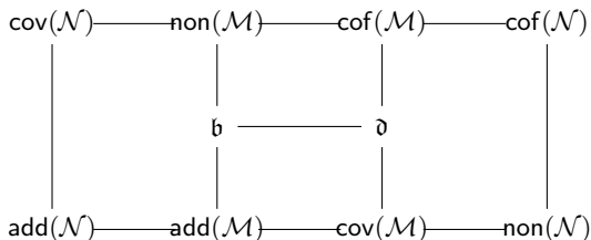
Fig. 0. Cichoń’s diagram
